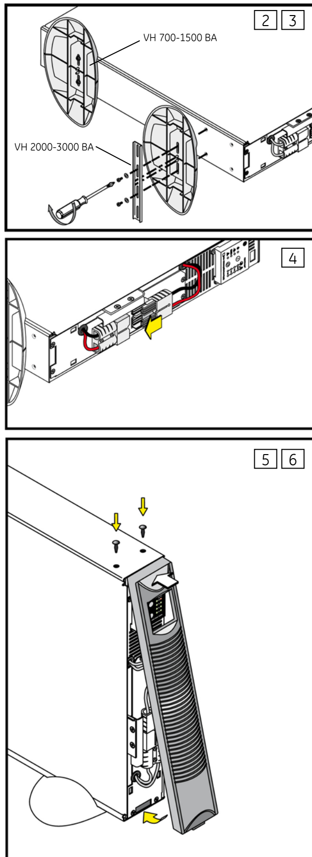
Рис. 3.3.1: Подготовка к вертикальной установке
