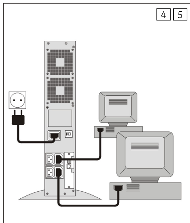
Рис. 3.6.2: Подключение электропитания к ИБП и нагрузке
